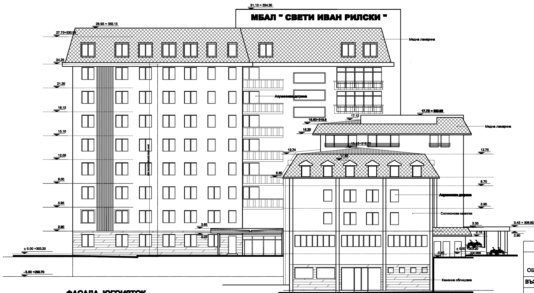
ФАСАДА ЮГОИЗТОК
