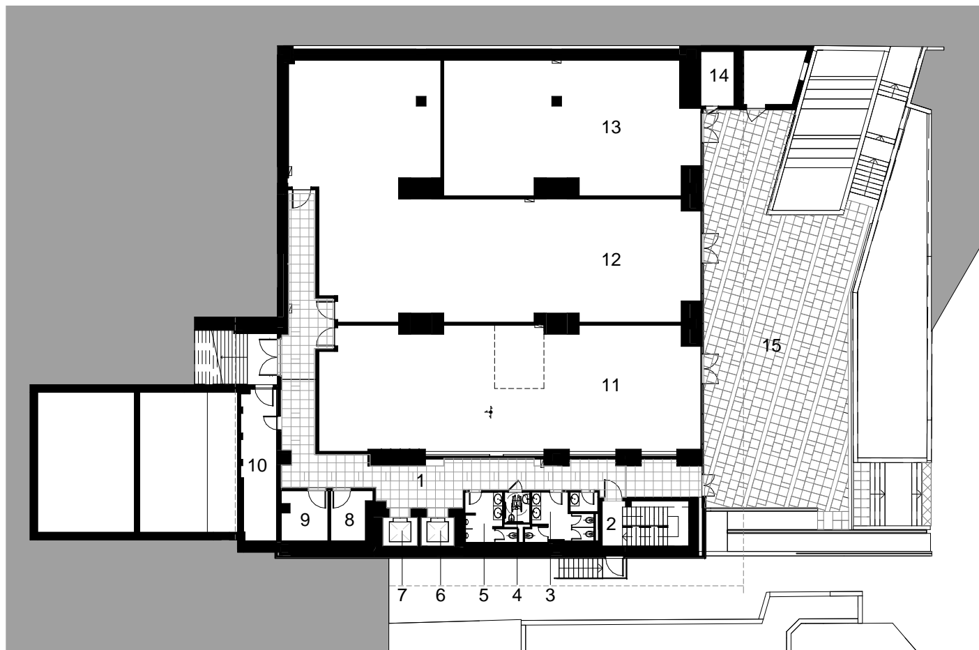
ПЛАН КОТА -3.60 / FLOOR PLAN, LEVEL -3.60
