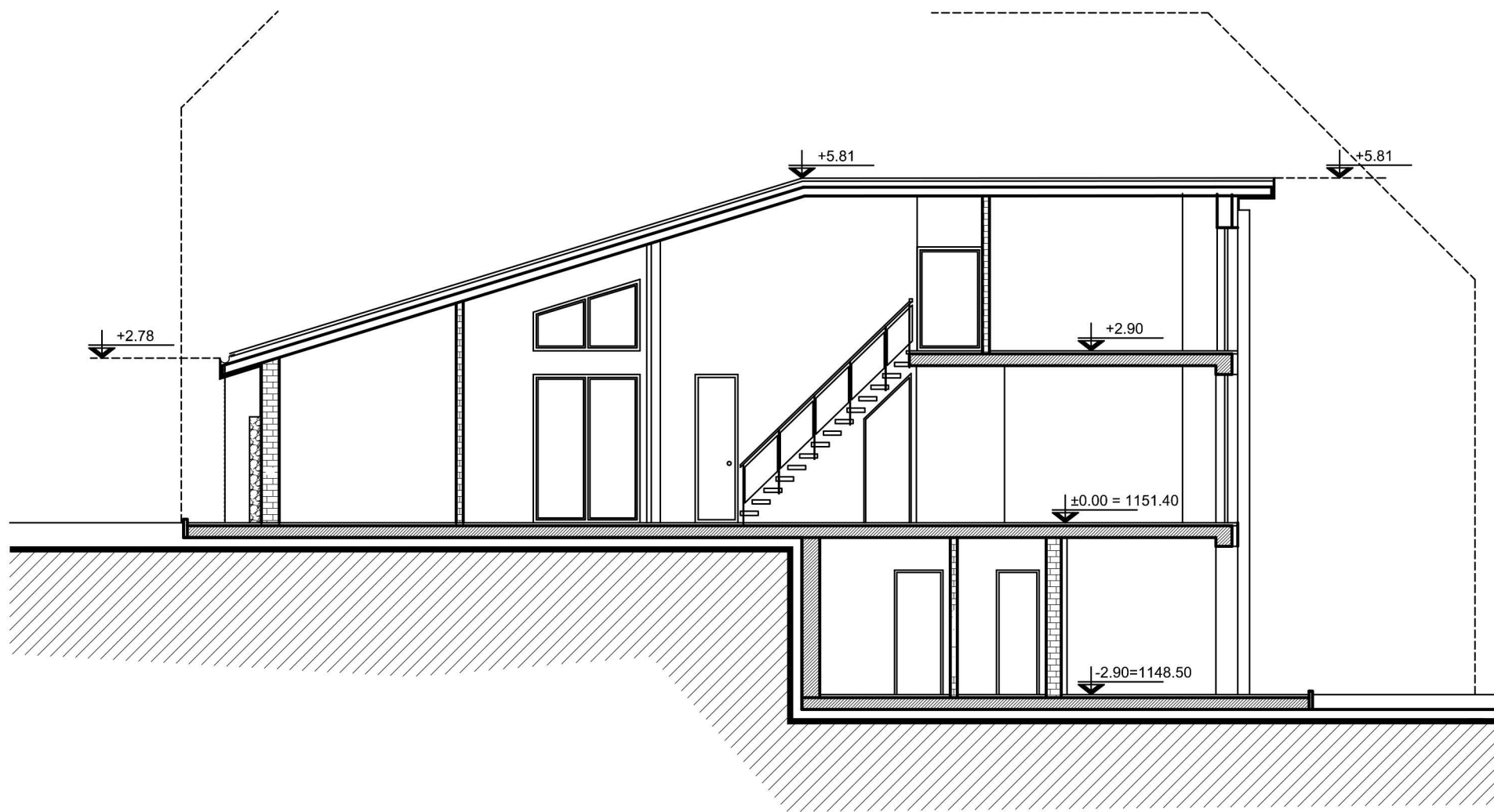
Разрез М 1:100
