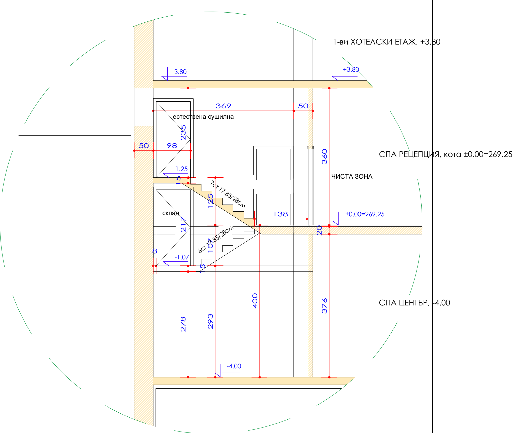
ЧАСТИЧЕН РАЗРЕЗ Г-Г М 1:50
