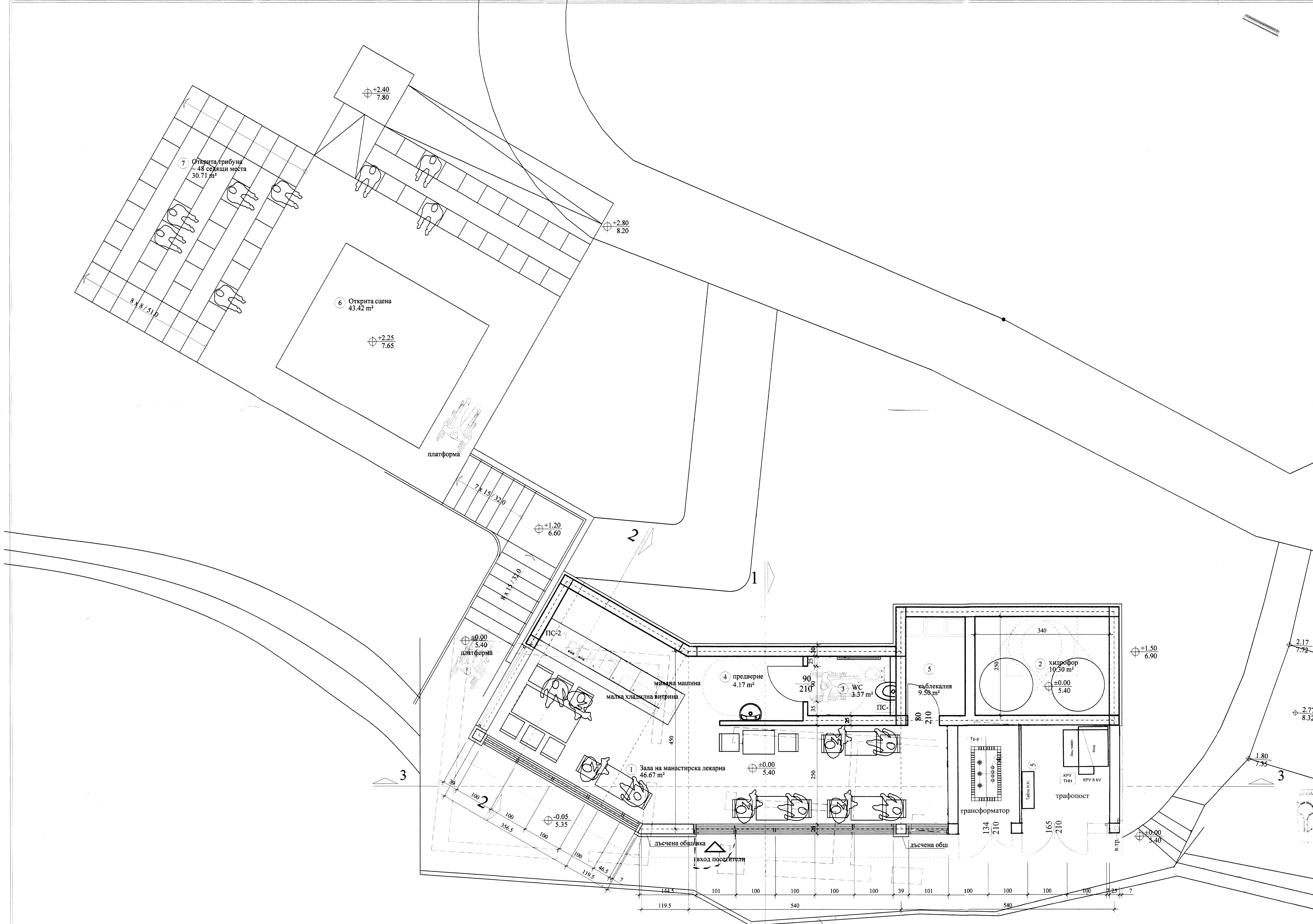
ПЛАН ПЪРВИ ЕТАЖ ЗП=83.14 м 2
