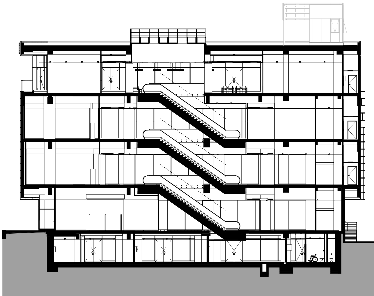
РАЗРЕЗ ПРЕЗ ЕСКАЛАТОРИТЕ / SECTION THROUGH THE ESPALATORS
