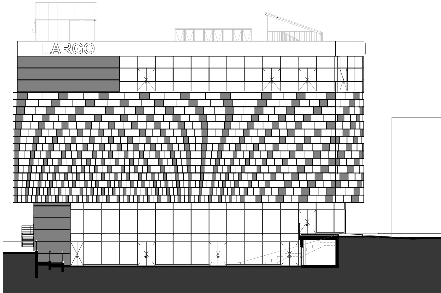
ФАСАДА КЪМ УЛИЦА "ТОДОР КАБЛЕШКОВ" / TODOR KABLESHKOV STREET ELEVATION
