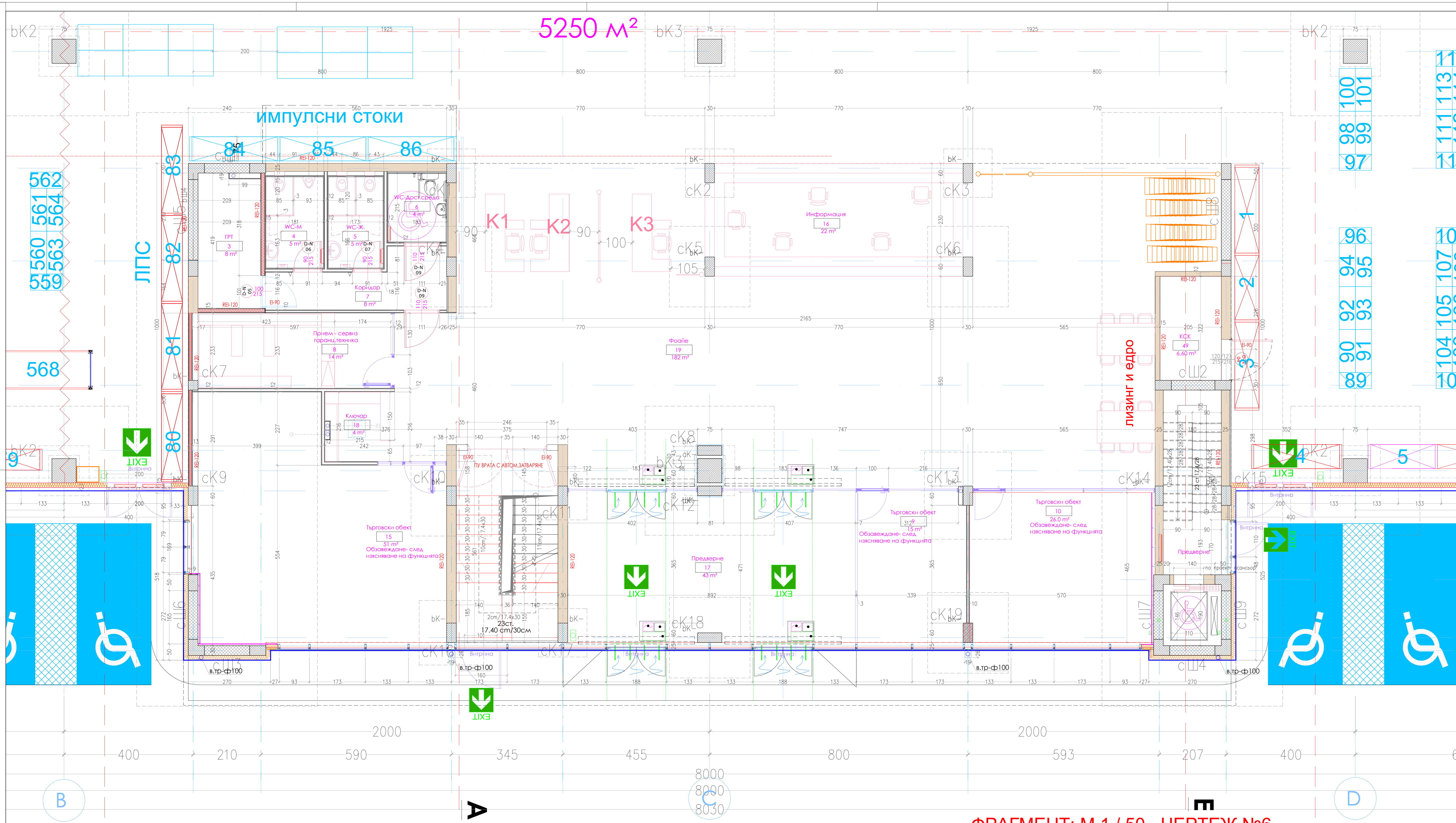
ФРАГМЕНТ: М 1 / 50 - ЧЕРТЕЖ №6
