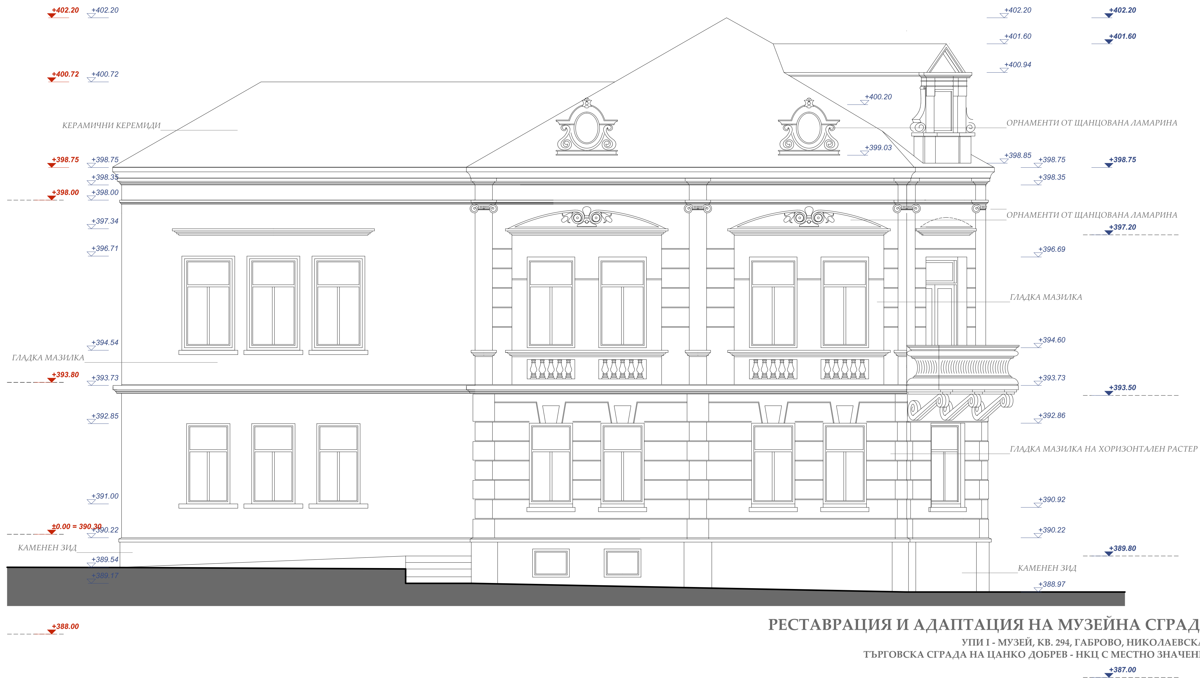
ФАСАДА СЕВЕР М 1 : 50
