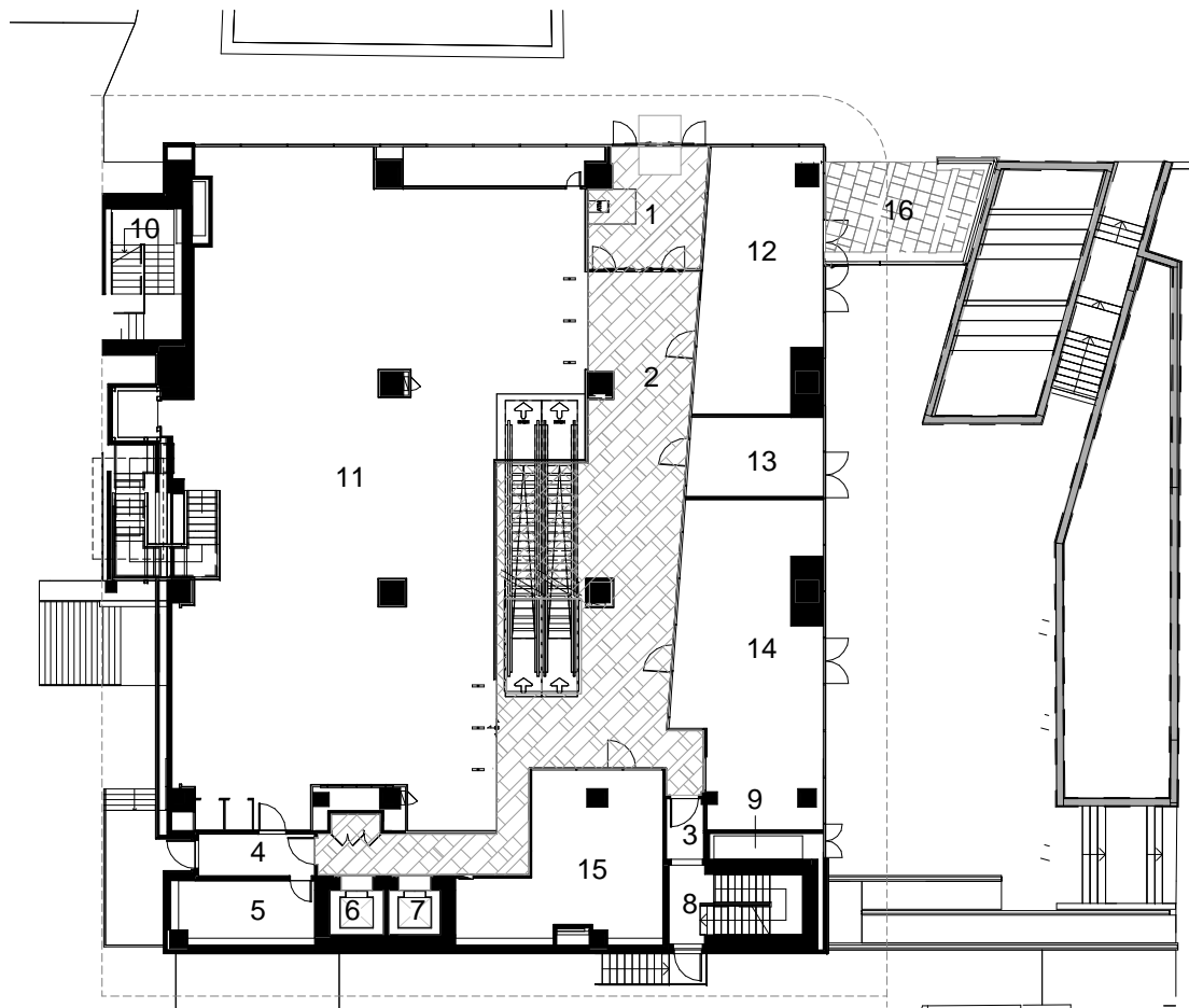
ПЛАН КОТА ±0.00 / FLOOR PLAN, LEVEL ±0.00
